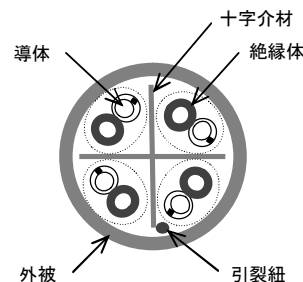
図1 断面構造
